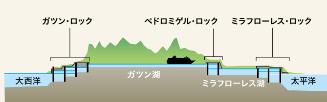
▶ パナマ運河断面
